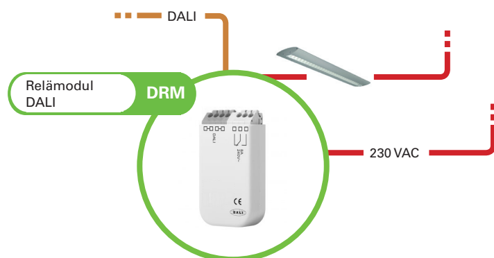
Anslutningsschema DRM.
