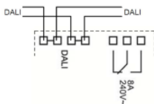
DRM – Inkopplingsplint DALI och brytspänning.
