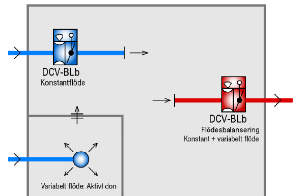
Konstantflödesstyrning med DCV-BLb.
