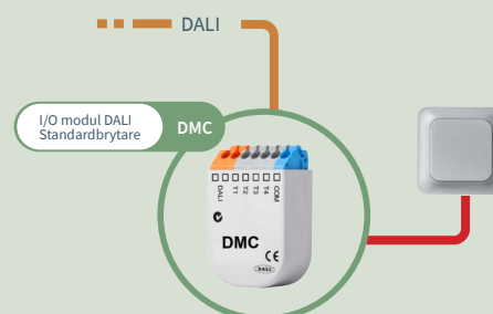
Anslutningsschema
