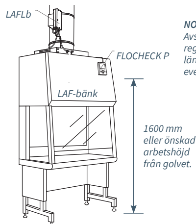
Illustration M1. Flocheck P monterad på LAF-bänk.
