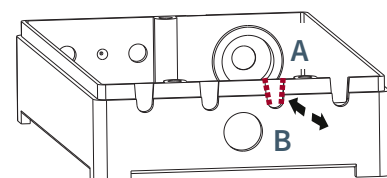
A: Klipp B: Vik fram och tillbaka/bryt av (Klipp/rensa uttag med avbitare)
