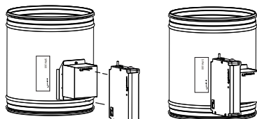
Spjällmotor med regulator monterade på det cirkulära spjället SPM.
