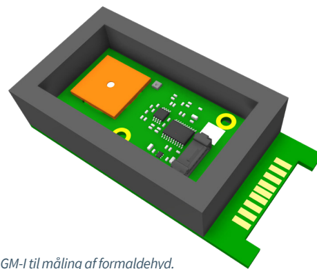
Udvidelseskort GM-I til måling af formaldehyd.
