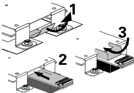
Montering af GM-I på pladsen for udvidelsesmodul på indersiden af spredelåget til ISQ og ISQ-F.
