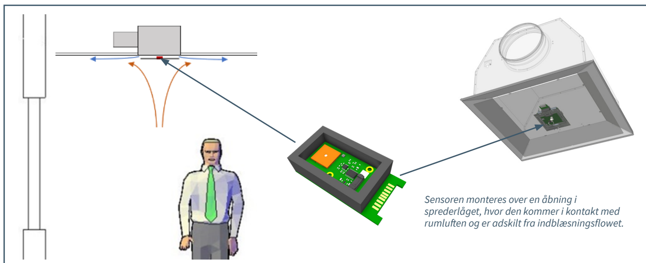
Udvidelseskort GM-I til måling af formaldehyd med placering i ISQ på indersiden af spredelåget.
