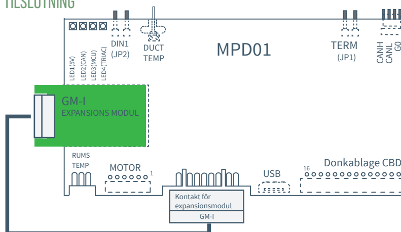
Sektion, der viser tilslutning af GM-I til stikket for udvidelseskort under kredsløbskortholderen på spredelåget til ISQ.
