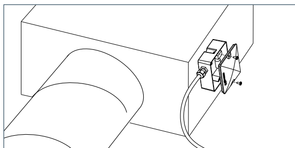
GT-D eller GTN-D montage på frånluftsdon.
