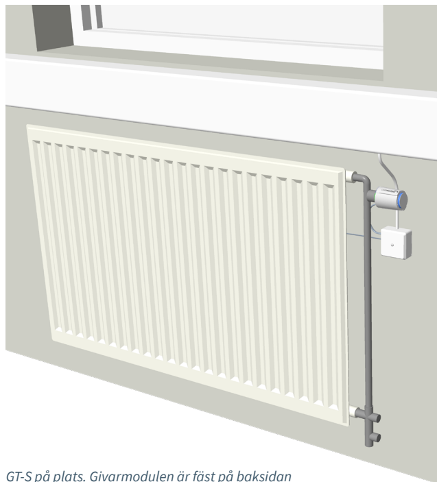
GT-S på plats. Givarmodulen är fäst på baksidan av radiatoren, ventilställdonet är monterat på radiatorventilen och anslutningsboxen är fäst på väggen med ansluten 4-ledare till rumsklimatsregulatorn.
