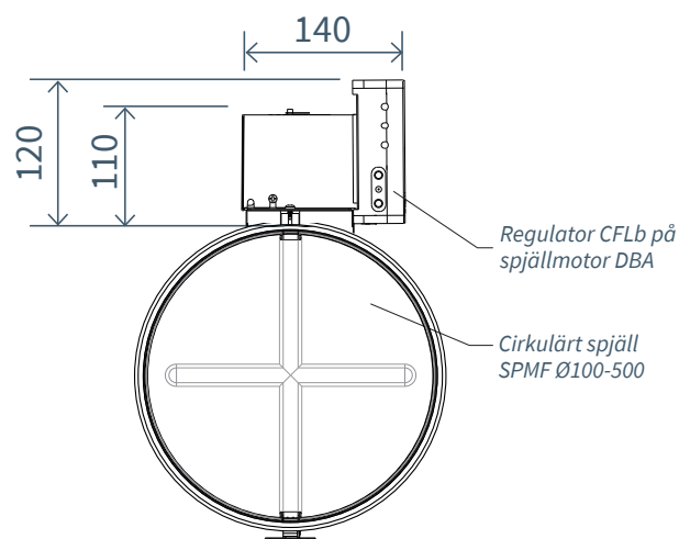
Byggmått för DCV-CFb Cirkulär.
