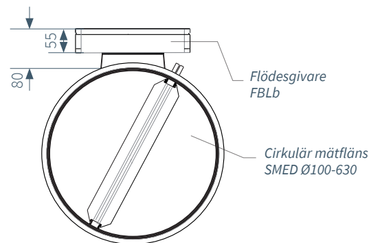
Byggmått för DCV-MFb Cirkulär.
