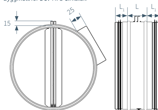
Mätfläns SMED med mått.
