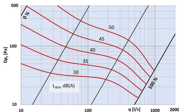
Diagram 7: Total A-vägd ljudefektnivå, dB(A) för SPMF-400
