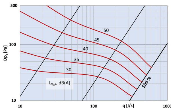
Diagram 6: Total A-vägd ljudefektnivå, dB(A) för SPMF-315
