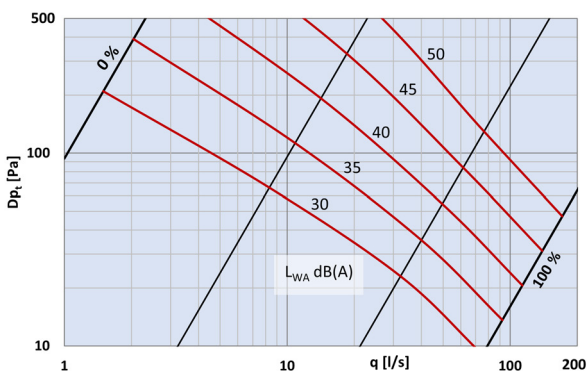
Diagram 3: Total A-vägd ljudefektnivå, dB(A) för SPMF-160
