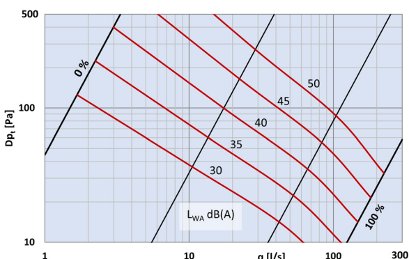
Diagram 4: Total A-vägd ljudefektnivå, dB(A) för SPMF-200
