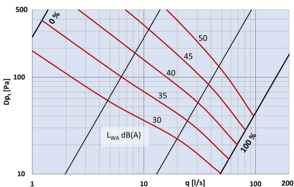
Diagram 2: Total A-vägd ljudefektnivå, dB(A) för SPMF-125
