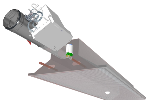
DCV-B på tilluftskanalen framför kylbaffeln med rumstemperatur- och närvarosensor GTO-B monterad på kylbaffelns raster.
