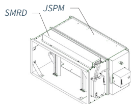
Illustration 1M. Montage av spjällmotor och regulator.
