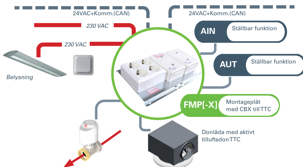
Anslutningsschema till FMP[-X].
