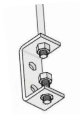
Exempel med ett U-beslag som upphängningsanordning. Beslaget monteras på ovansidan med skruv (M8x16).
