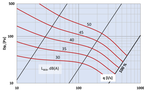
Diagram 6: Total A-vägd ljudeffektnivå, dB(A) for SPMF-315
