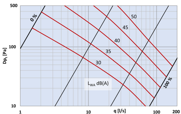
Diagram 3: Total A-vägd ljudeffektnivå, dB(A) för SPMF-160
