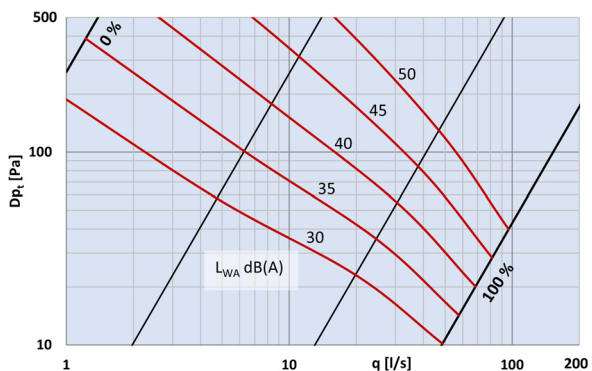
Diagram 2: Total A-vägd ljudeffektnivå, dB(A) för SPMF-125
