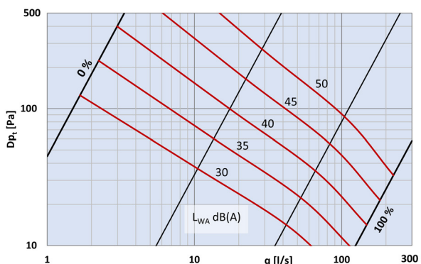
Diagram 4: Total A-vägd ljudeffektnivå, dB(A) för SPMF-200
