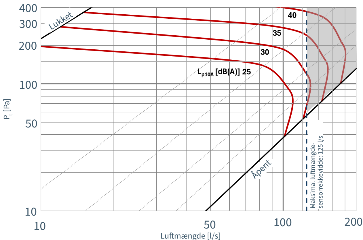
Diagram ICI-F-200, Lydtrykniveau L_{P10A} dB(A)
