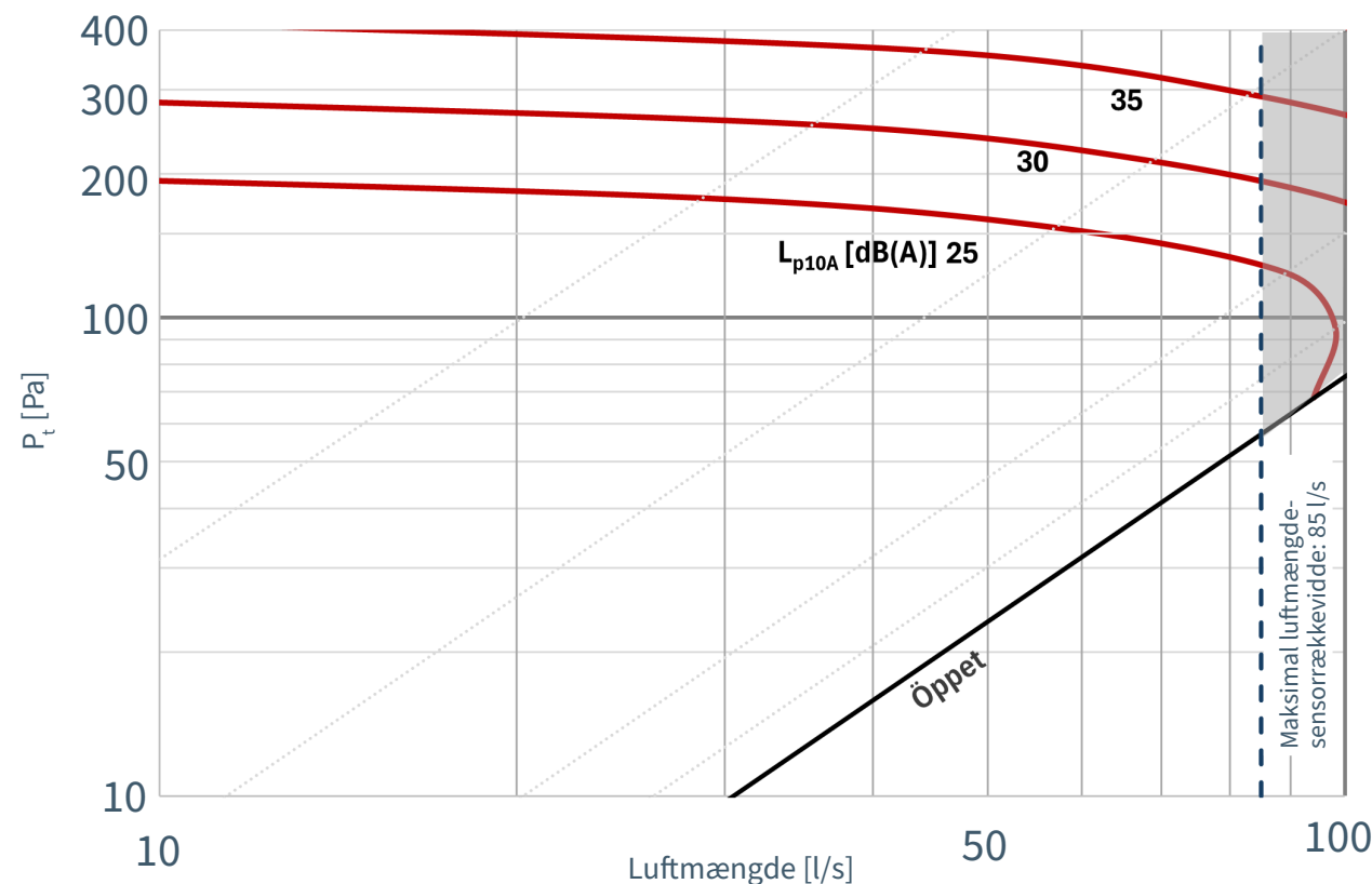
Diagram ICI-F-160, Lydtrykniveau L_{P10A} dB(A)
