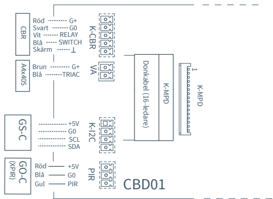
Sektion av kretskort i kopplingsbox CBD. GS-C kopplas in via K-I2C.
