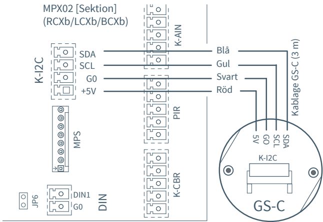
Sektion av kretskort till rumsklimatsregulatorer med plint K-I2C för inkoppling av GS-C.
