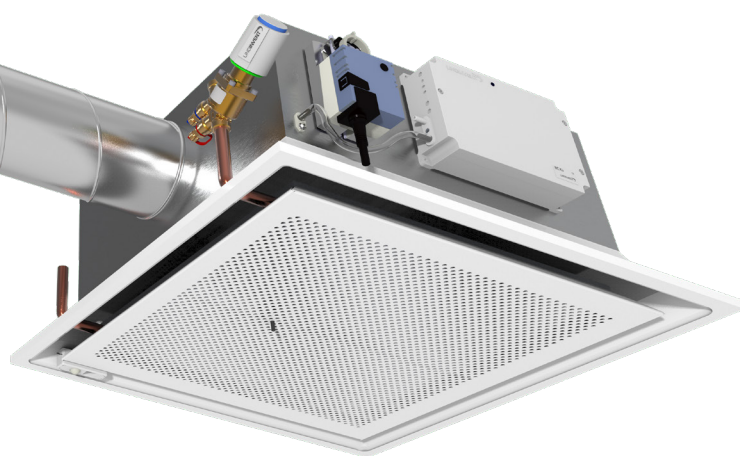
VAV-baffel utrustad med BCXb, sensorna BSX och BST
